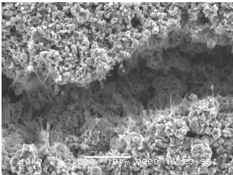
VGCF 碳管在正極材料中之分散圖
