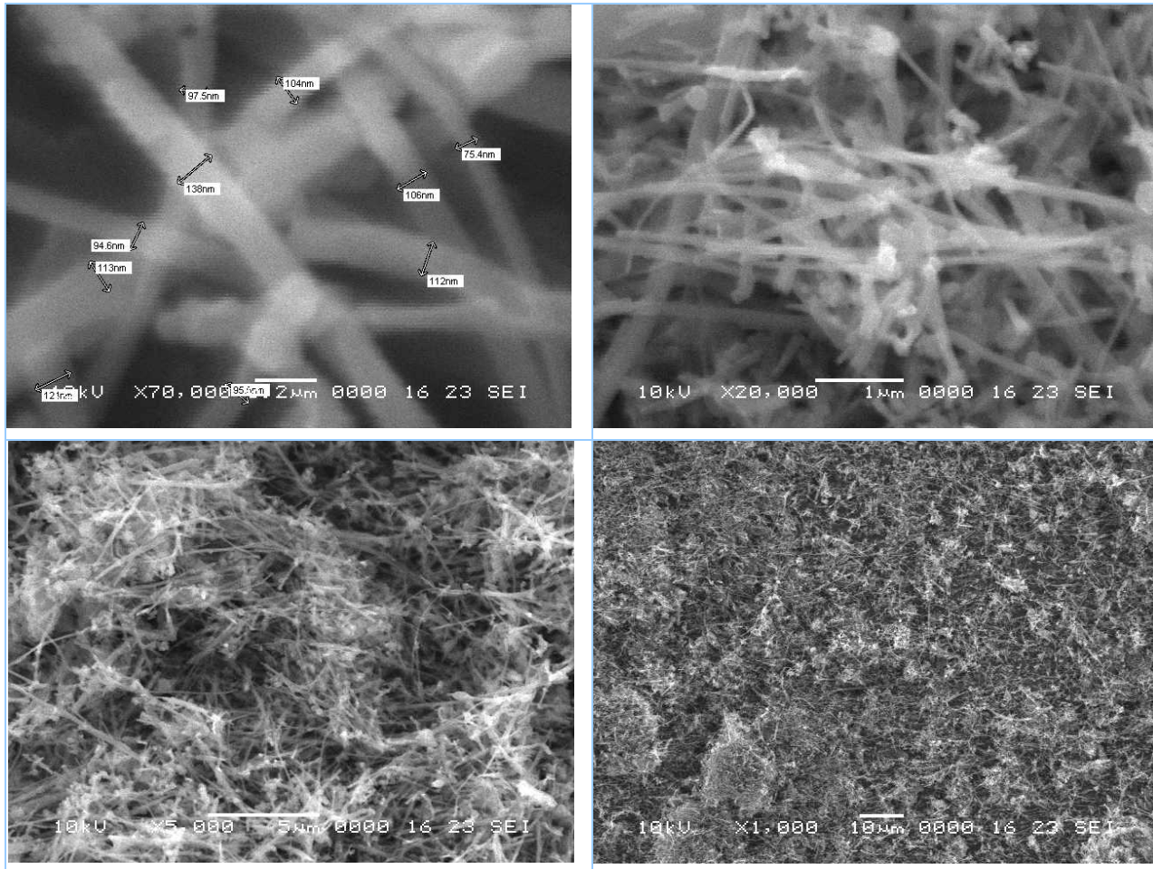
VGCF 碳管在正極材料中之分散圖
